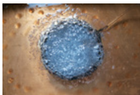
Provozdušňování chladicího a mazacího prostředku
